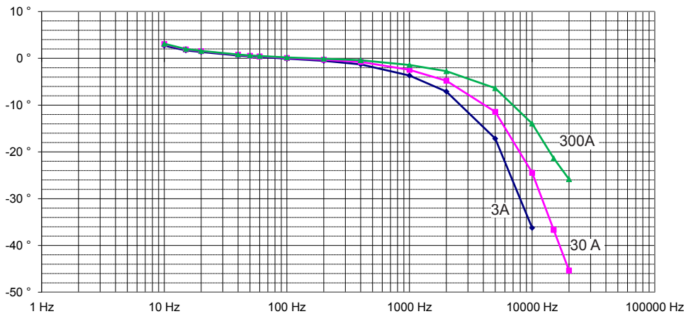
Enfas mätområde 3 A, 30 A och 300 A
