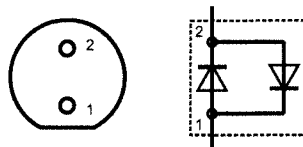
LED-Anschluß
