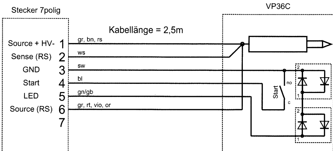
LED-Anschluß
