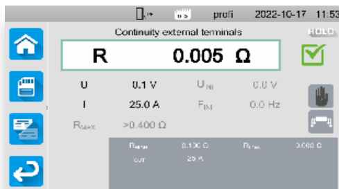
Tulosnäyttö yksityiskohtaisessa näyttötilassa: Jatkuvuuden mittaus 25 A:n virralla, 4-johdinkytentä (CA 6163)
