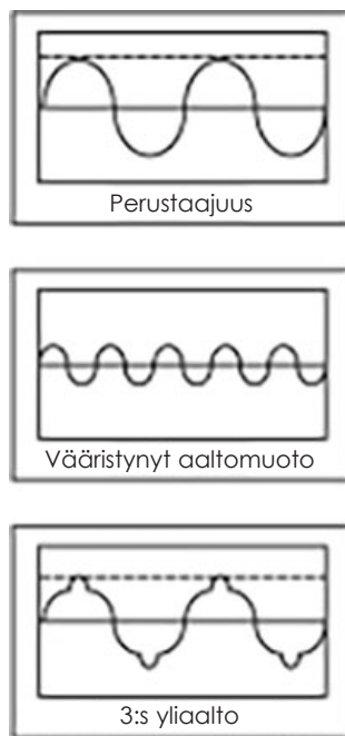
Kuva 13: Perustaajuus + kolmas yliaalto
