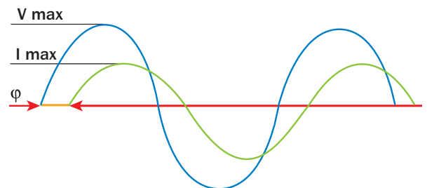
Kuva 2: Jännitteen ja virran välinen vaihesiirtymä
