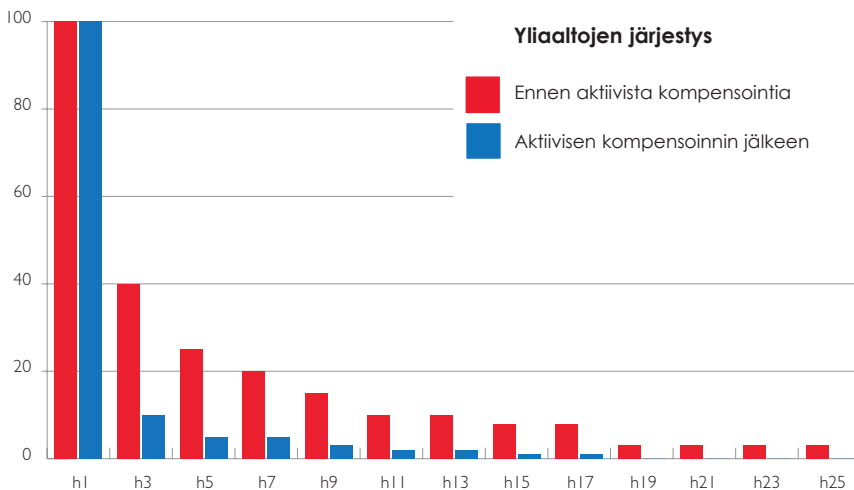
Kuva 17: Yliaaltospektri näyttää tyypillisen tilanteen ennen ja jälkeen aktiivisen yliaaltosuodattimen asennusta. Tämä parannettu spektri antaa myös parempia käyrämuotoja sekä jännitelle että virralle.
