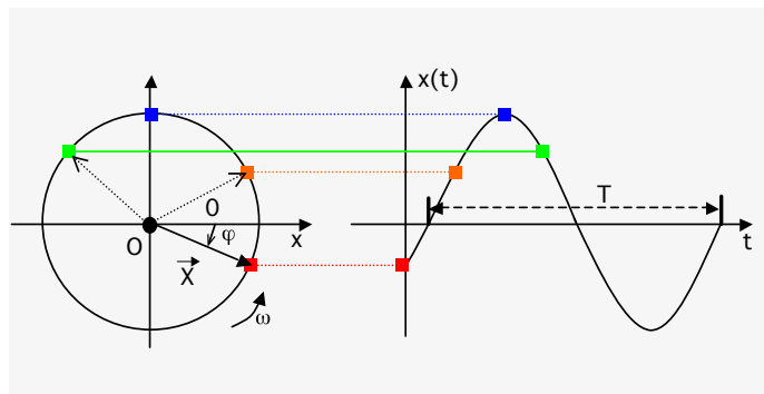
Kuva 8: Vektorin \vec{X} ja signaalin x(t) välinen suhde
